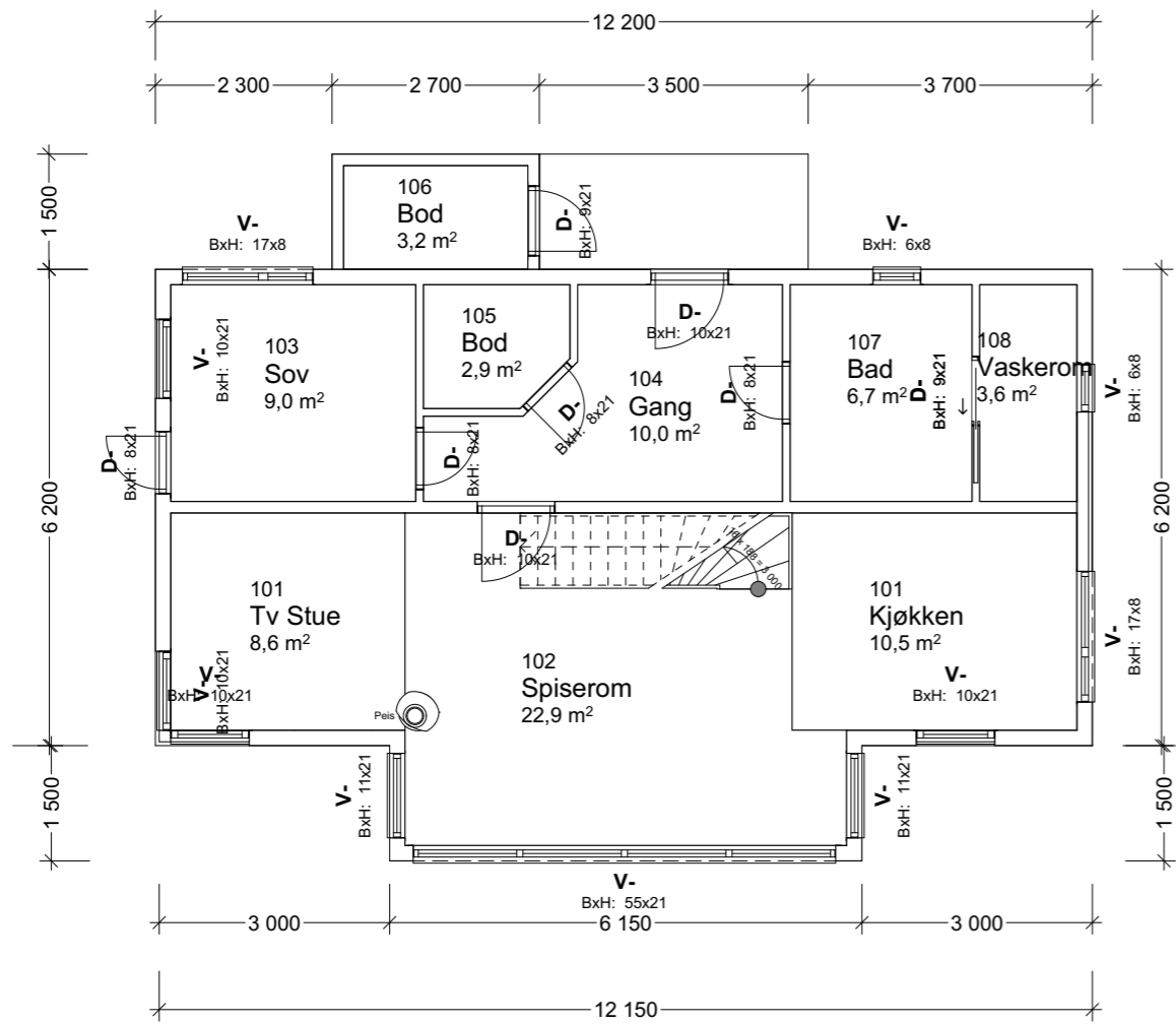
Plan 1. etasje
